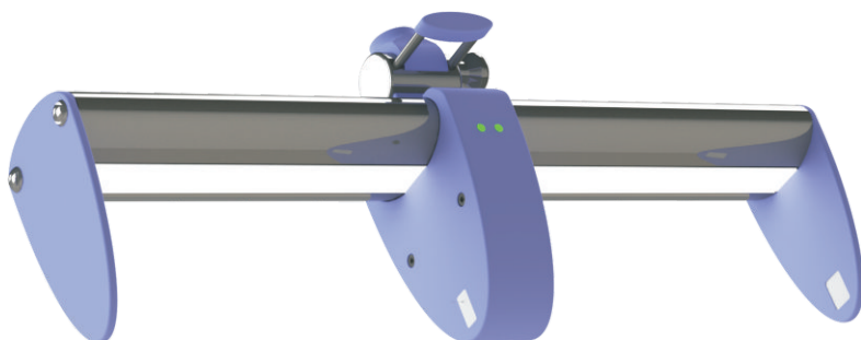
PPL-Ovali-500 LS1 LED-Prüfplatzbeleuchtung mit Lichtschrankenmodul 1-strahlig (Rotlicht) Objekterkennung 90 mm senkrecht zur Lichtaustrittsfläche LED- Anzeige Links-Rechts
