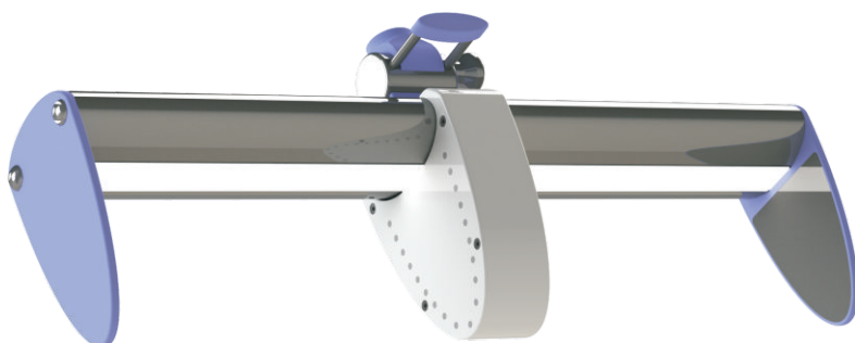
PPL-Ovali-500 LSE LED-Prüfplatzbeleuchtung mit Lichtschrankengitter Infrarot (nicht sichtbares Licht) elliptische, umlaufende Lichtgitteranordnung Objekterkennung von 0 - 100 mm von Lichtaustrittsfläche LED- Anzeige Links-Rechts
